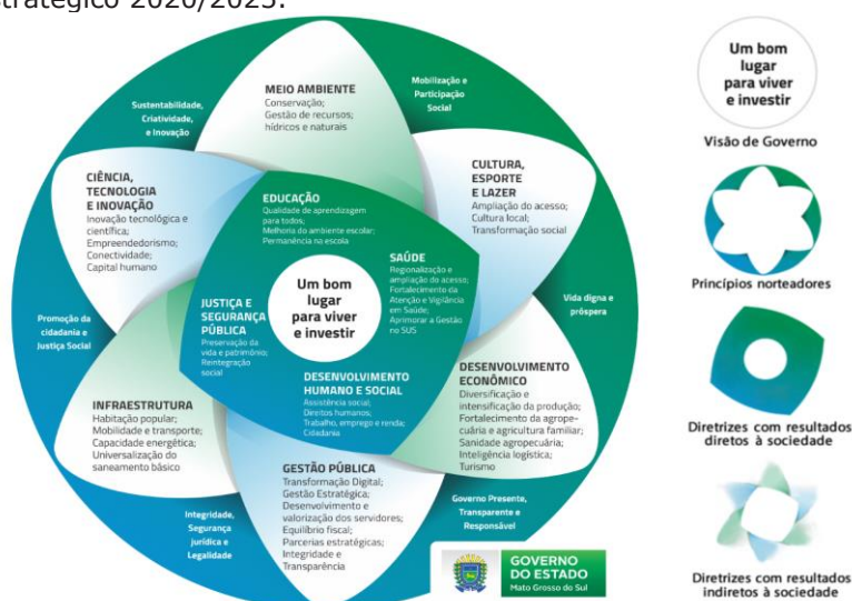
Figura 03: Mapa Estratégico 2020/2023.
