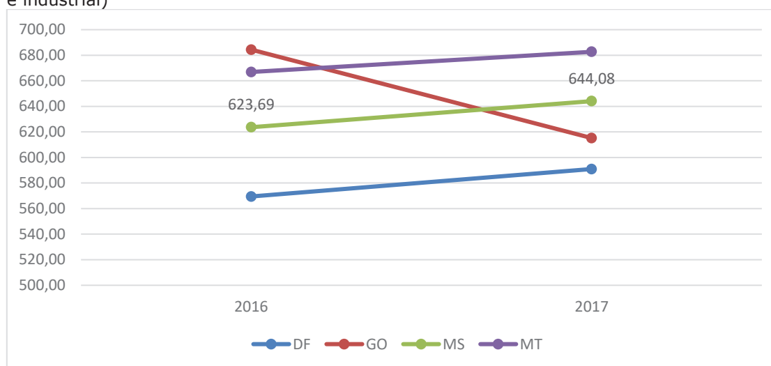
Gráfico 27 – Custo da Energia Elétrica (tarifa média praticada (R$/MWh) para o consumo comercial, residencial e industrial)
