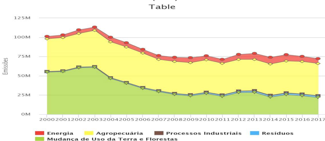
Gráfico 26 - Emissões de CO2 em toneladas (SEEG).
