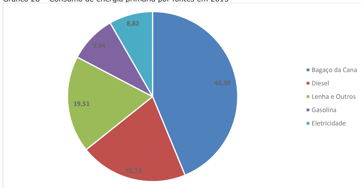
Gráfico 28 – Consumo de energia primária por fontes em 2015
